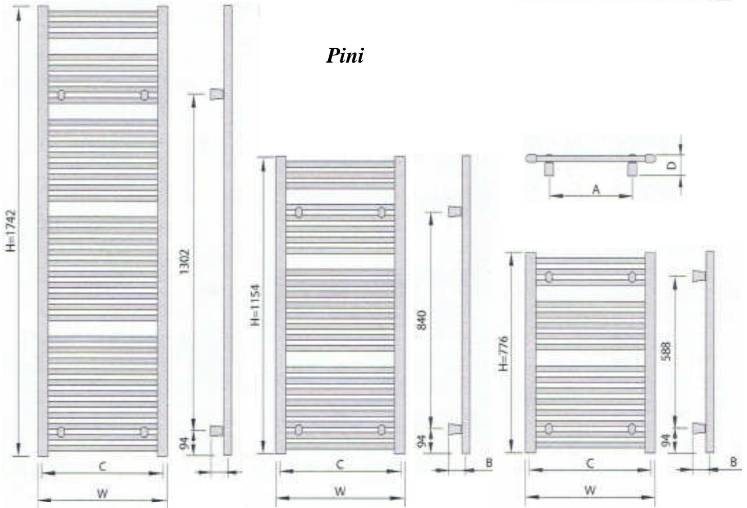
Höjd 1742 mm
